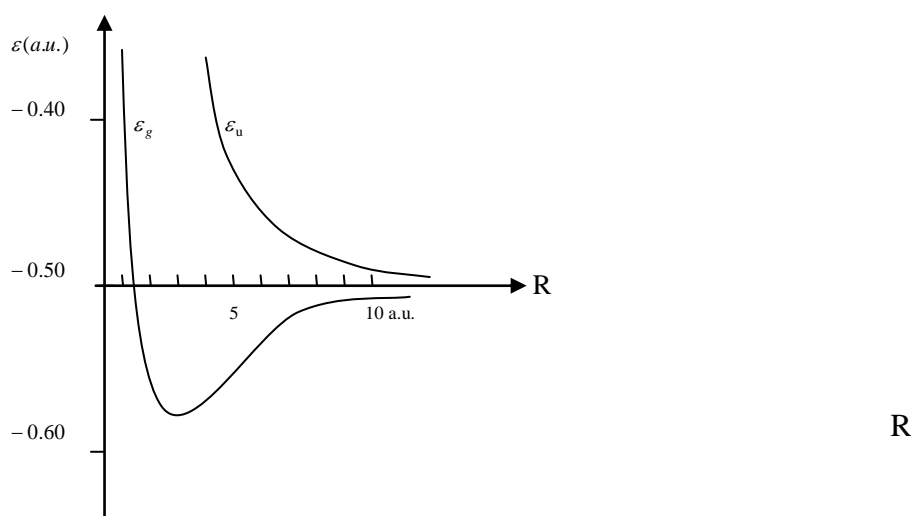
ل (2.2) - انرژی کل یون که تابعی از فاصله بستگی برای در حالت و است رسم نشده (واحد ها، واحدهای اتمی هستند).
