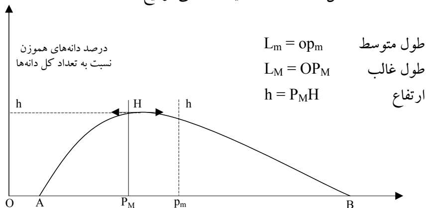
شکل ۵- حالت کلاسیک منحنی توزیع های آماری
